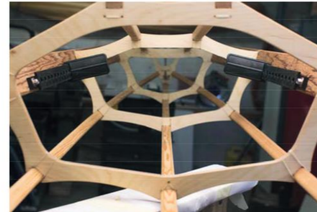
2 - Eingebaute Fußstützen
